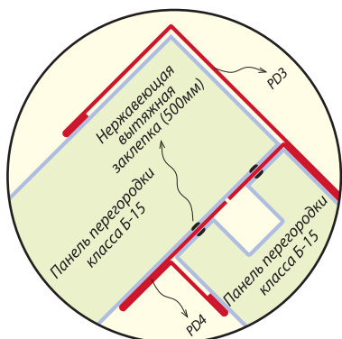
Угловая деталь
