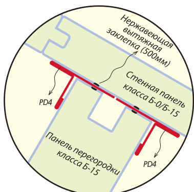
Деталь соединения-1
