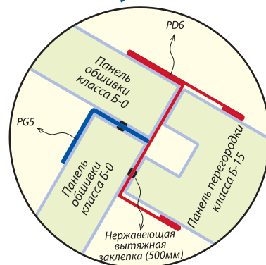
Наружная угловая деталь установки
