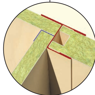
Вертикальная секция установки
