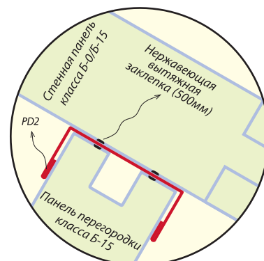
Деталь соединения-2
